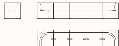
Congif. 16 367.112.Z93.B16 OW 3600mm OD 720mm OH 720mm SH 400mm
