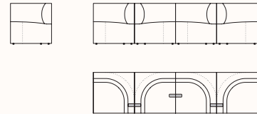
Congif. 5 367.112.Z5.B5 OW 2880mm OD 720mm OH 720mm SH 400mm
