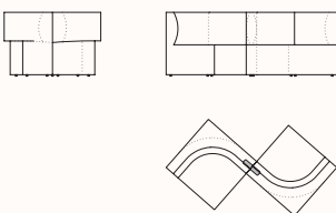
Congif. 6 367.112.V.B6 OW 1910mm OD 1080mm OH 720mm SH 400mm
