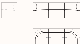
Congif. 14 367.112.Q.B14 OW 2160mm OD 720mm OH 720mm SH 400mm
