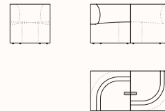
Congif. 7 367.112.Q.B7 OW 1440mm OD 720mm OH 720mm SH 400mm
