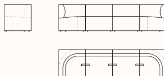
Congif. 15 367.112.Z5.B15 OW 2880mm OD 720mm OH 720mm SH 400mm
