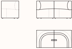
Congif. 1 367.112.Q.B1 OW 1440mm OD 720mm OH 720mm SH 400mm
