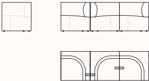
Congif. 3 367.112.X.B3 OW 2160mm OD 720mm OH 720mm SH 400mm
