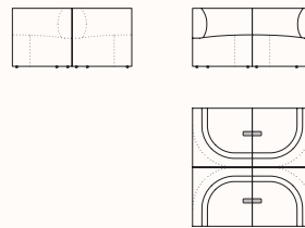
Congif. 12 367.112.QQ.B12 OW 1440mm OD 1440mm OH 720mm SH 400mm
