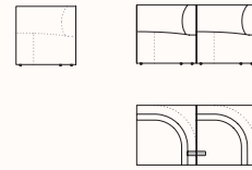
Congif. 10 367.112.Q.B10 OW 1440mm OD 720mm OH 720mm SH 400mm
