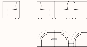
Congif. 4 367.112.X.B4 OW 2160mm OD 720mm OH 720mm SH 400mm
